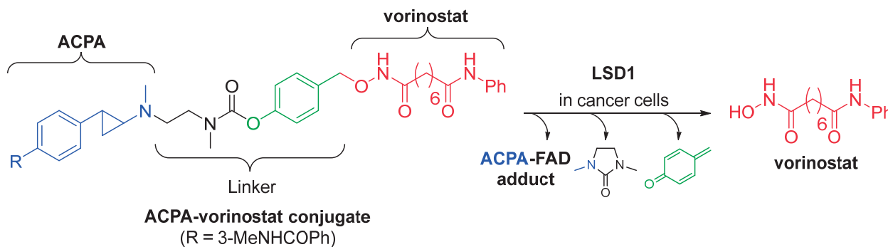
がん細胞選択的に抗がん剤 vorinostat を放出する ACPA-vorinostat conjugate
