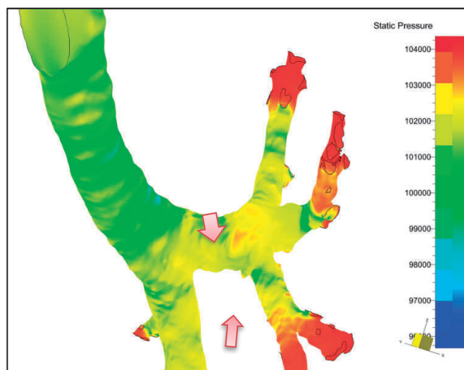
胸腔陽圧時に気道閉塞をきたした症例での流体力学 3 次元解析結果
